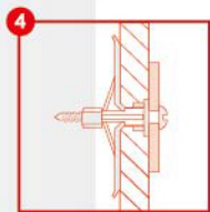
เมื่อจับตะปูเกลียวยึดเข้ากับพุกจนสุดแล้ว ปีกของพุกจะขยายออกและยึดแน่นกับแผ่นสมาร์ทบอร์ด
